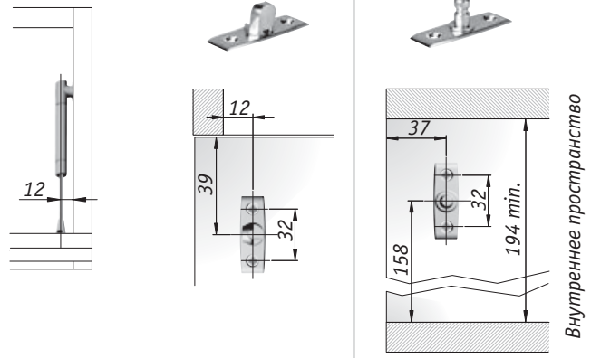
Использование креплений под саморез
