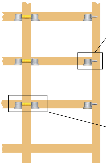
Вариант фиксации с саморезом
