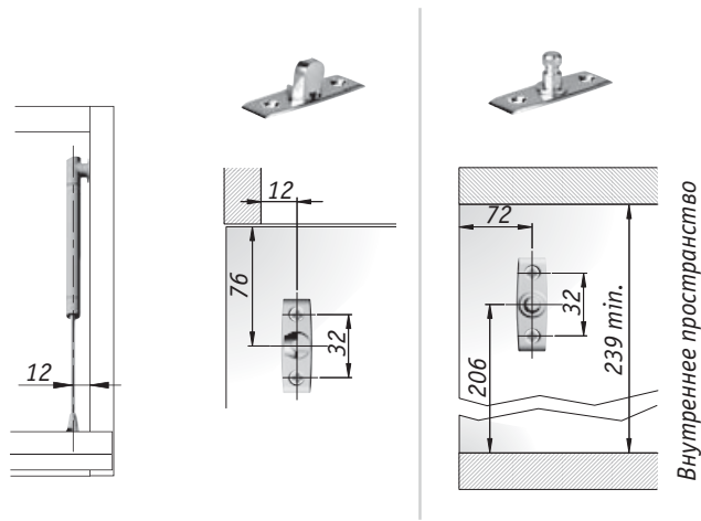
Использование креплений под саморез
