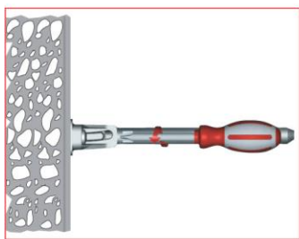
1. Ослабить фиксирующие саморезы
