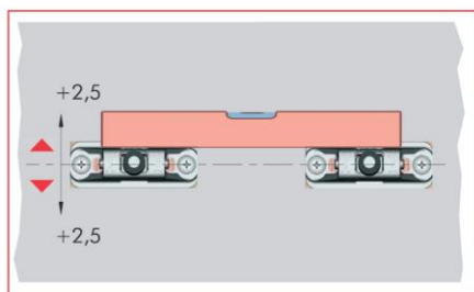
2. Отрегулировать крепления
